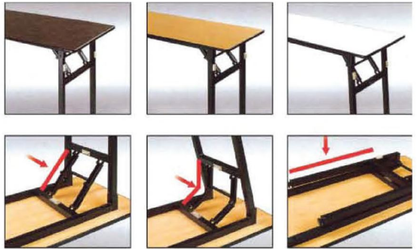
ขาล็อคสปริง แข็งแรงยิ่งกว่า Positive Locking Hinge
